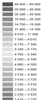
b) metoda Kriging Simple
