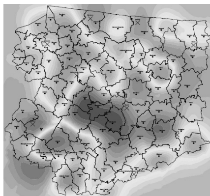
b) metoda Kriging Simple
