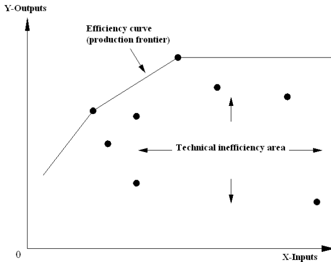
Rysunek 1. Krzywa efektywności ( best practice frontier )
